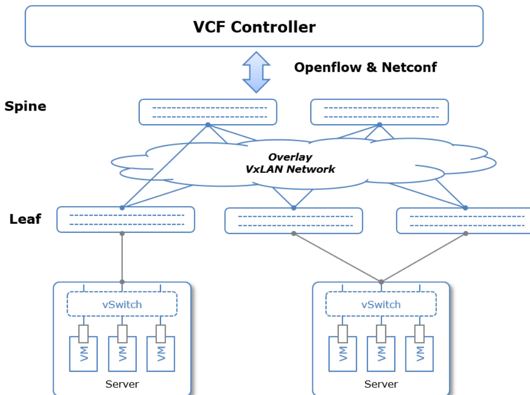
S9855 系列交换机在 Overlay 数据中心的应用
